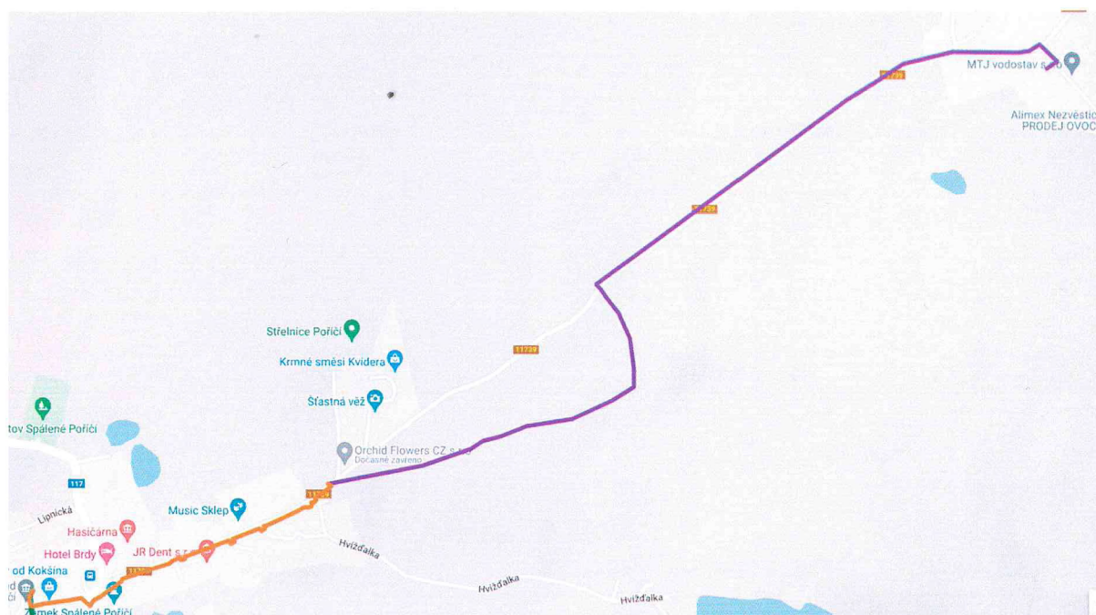
Obr.: Oranžová - intravilán města Spálené Poříčí (zafouknutí kabelu do stávající chráničky HDPE40), Fialová - nový samostatný výkop.
